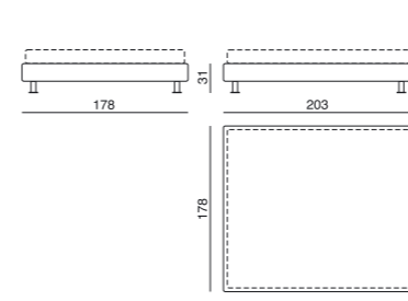
Letto matrimoniale
