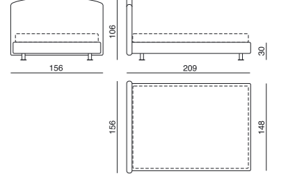
Letto francese
