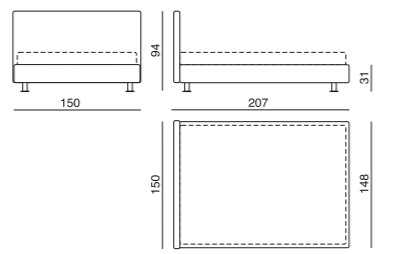
Letto francese
