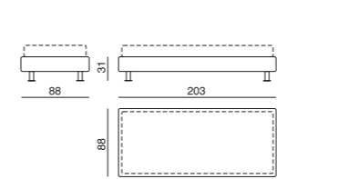
Letto singolo
