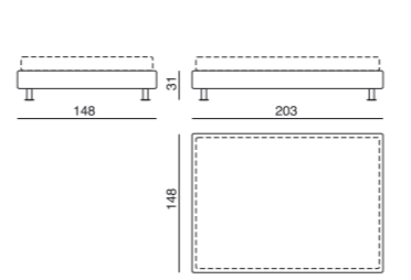
Letto francese
