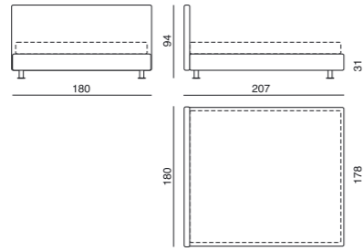
Letto matrimoniale
